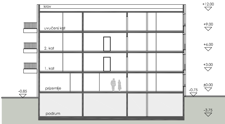
presjek 1-1 1:200
