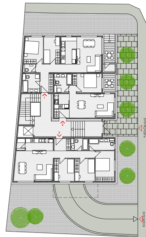
tlocrt prizemlja 1:200
