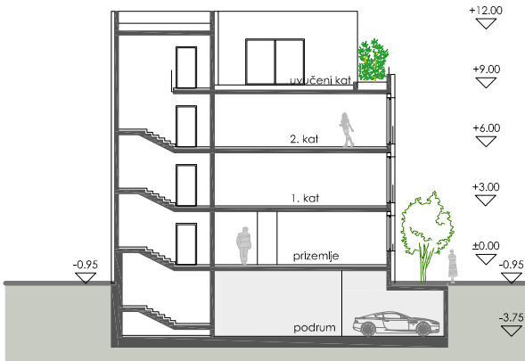
presjek 2-2 1:200
