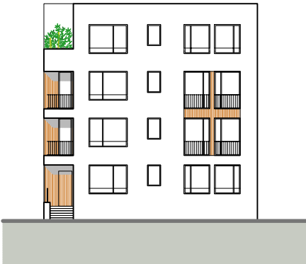
sjeverno pročelje 1:200
