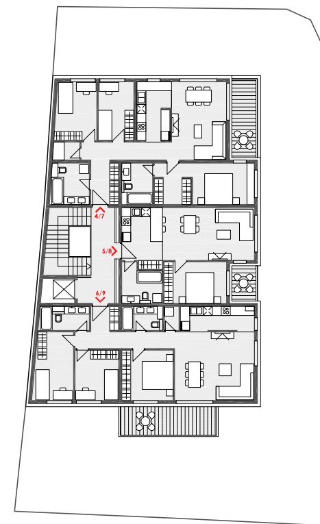
tlocrt 1./2. kata 1:200
