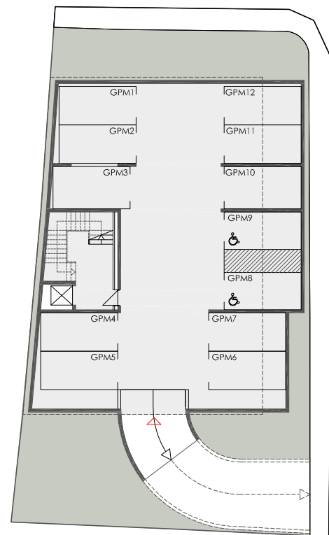
tlocrt podruma 1:200
