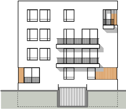
južno pročelje 1:200
