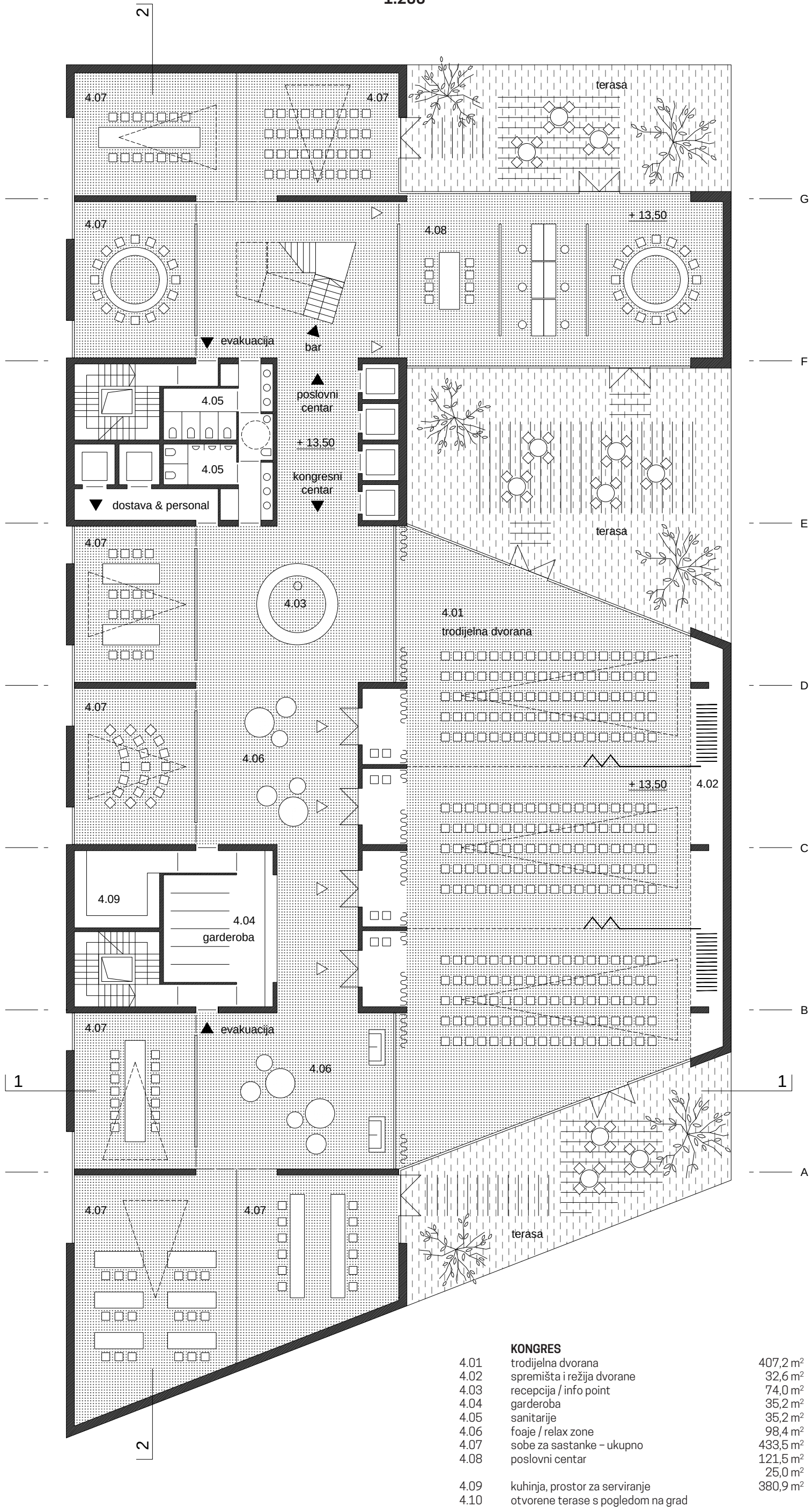
TLOCRT KONGRES +04 1:200
