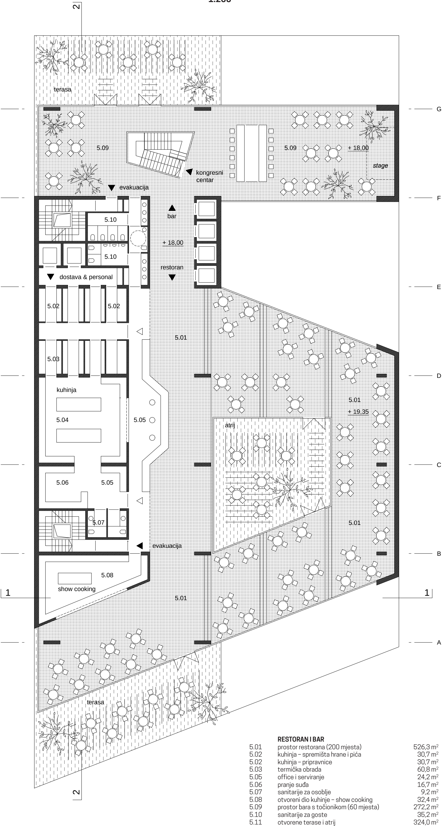
TLOCRT RESTORAN +05 1:200
